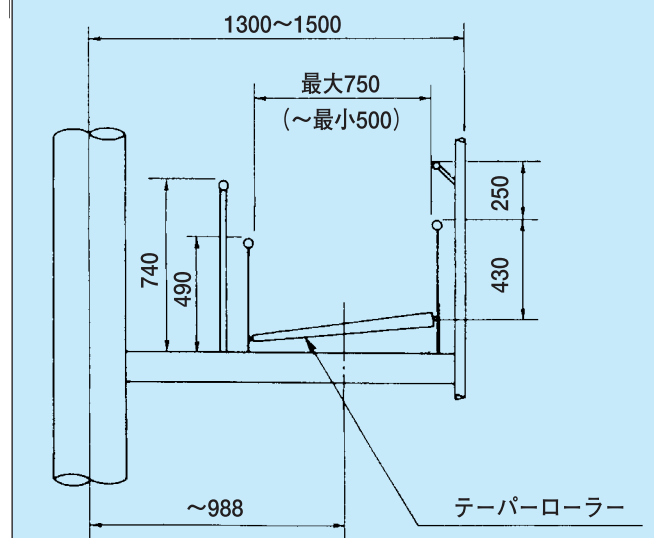
TR-型標準断面図
