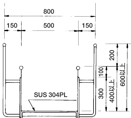
ST-型標準断面図
