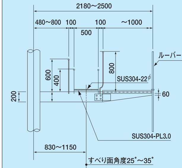
RS-型標準断面図
